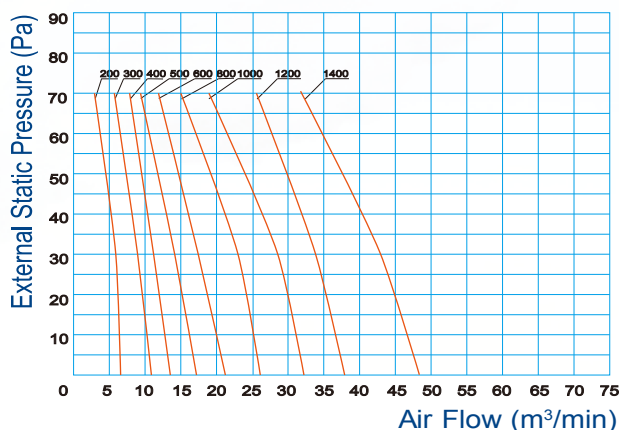
MKT4-200~1400G30
