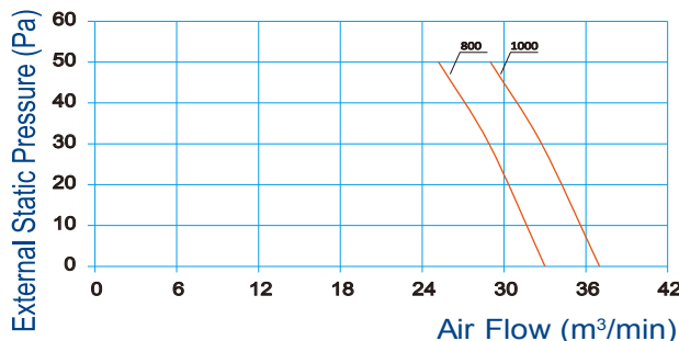
MKT3-800&1000G50-A4
